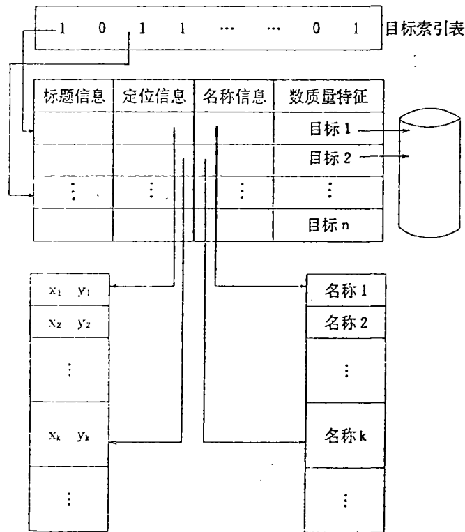
图4 目标数据库结构
