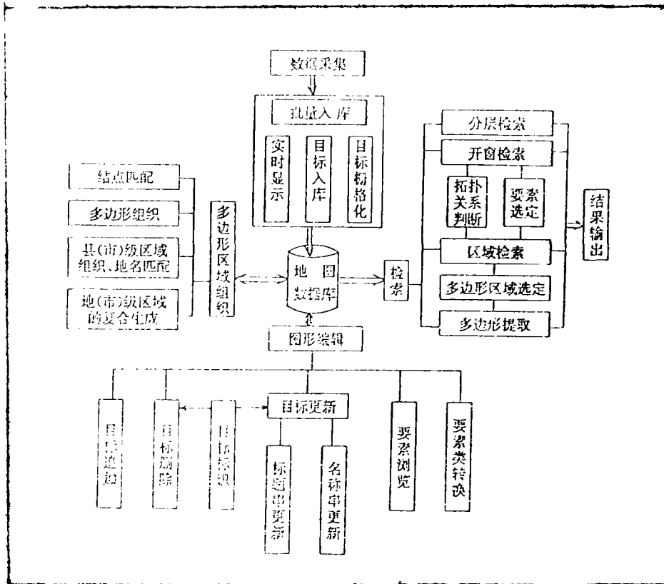
图 3 地理底图管理系统
