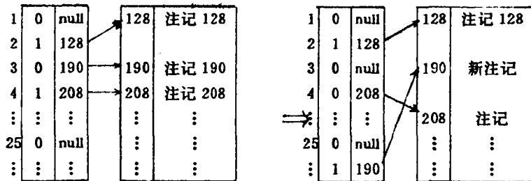
图4 目标数据库结构
